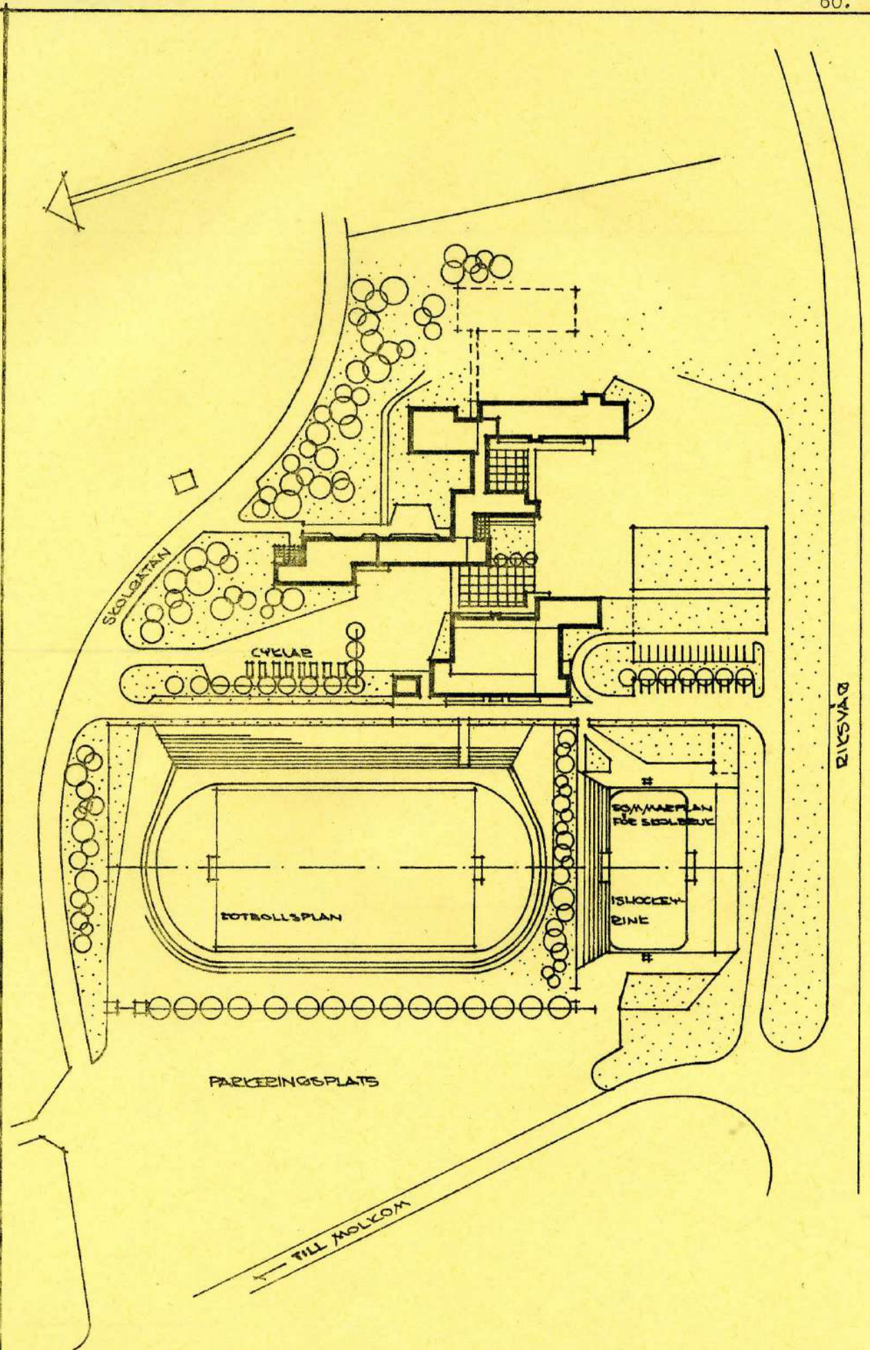
CENTRALSKOLA I MOLKOM ILLUSTRATIONSPLAN, SKALA 1:2000 ARK. SAR J. WÄSTLUNDSARKITEKTBYRÅ KARLSTAD 6-11-63
